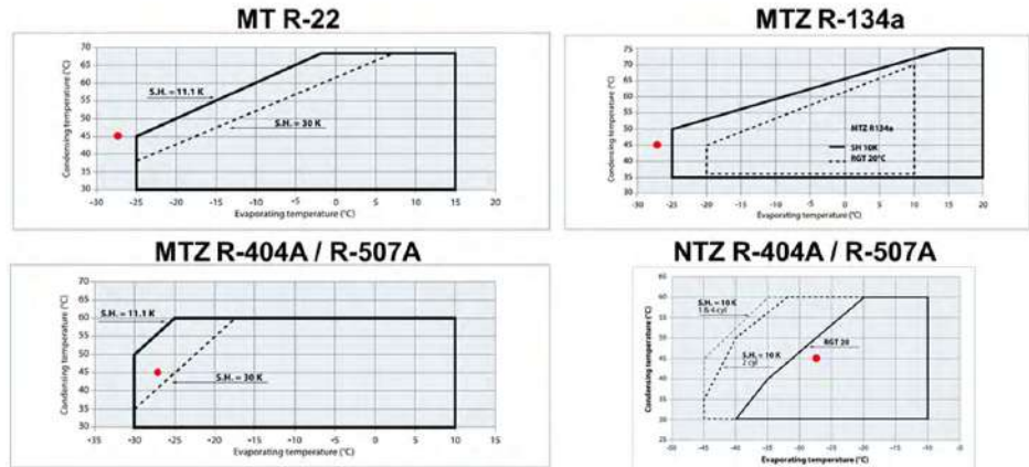
Imagen 75 Límites de aplicación de compresores Maneurop
