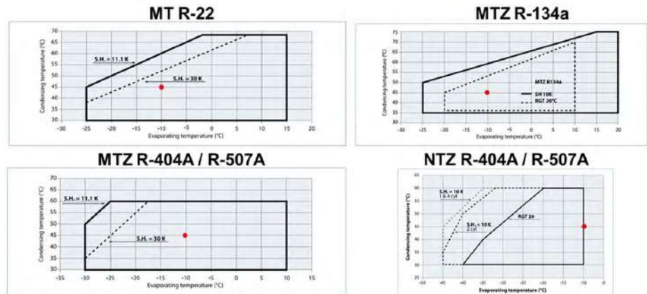
Imagen 76 Límites de aplicación de compresores Maneurop
