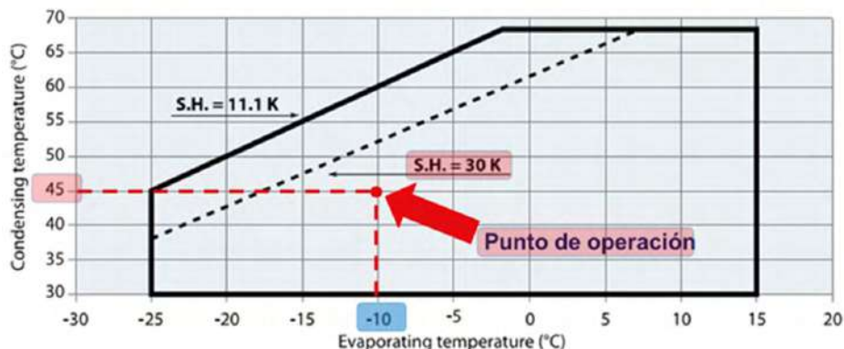
Imagen 73 Límites de aplicación de un compresor Maneurop MT utilizando R-22 Fuente: www.danfoss.com
